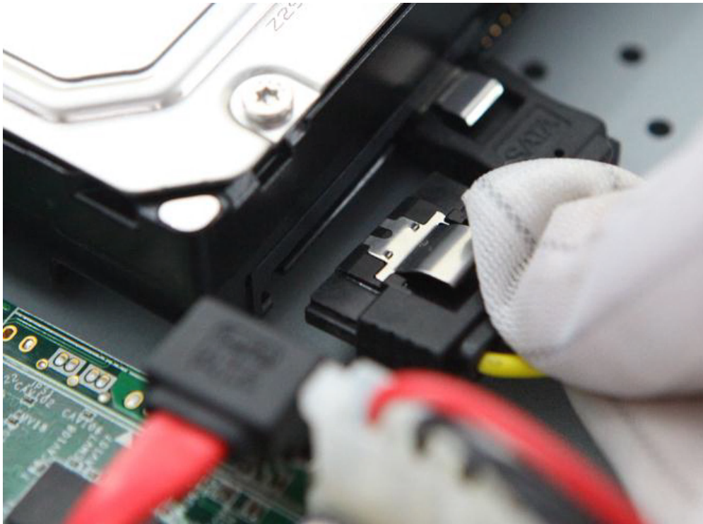
Cáp nguồn gắn trên ổ đĩa cứng
