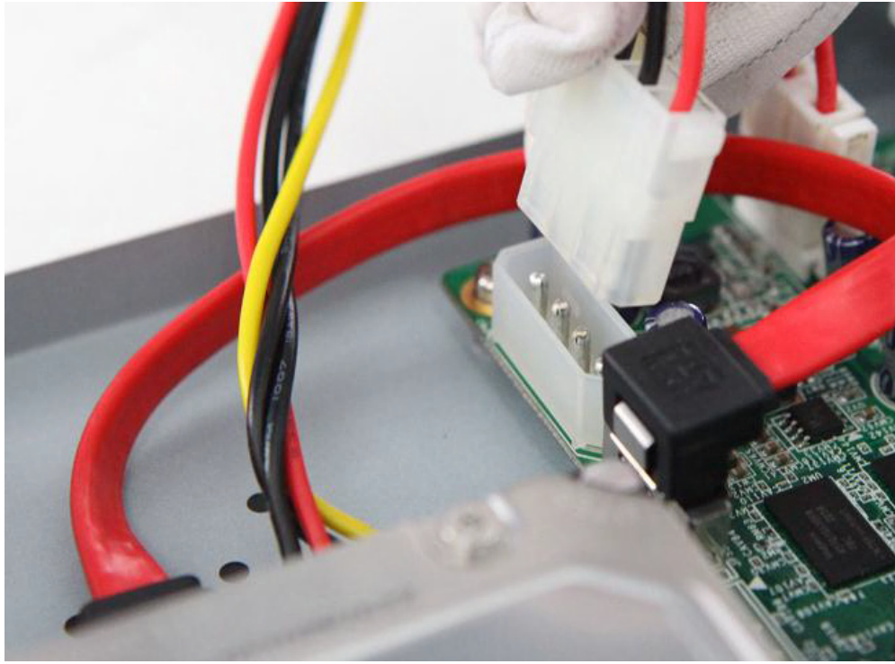
Cáp nguồn gắn trên board của đầu ghi
